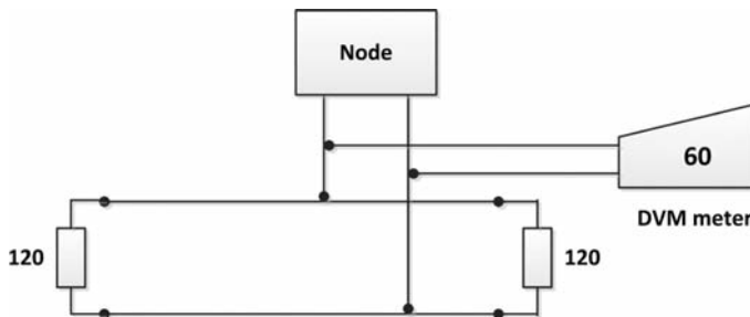
Slika 2.6 – Provera završetka linije
