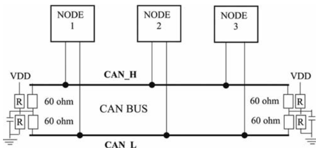
Slika 2.4 – Pristrasni podjeljeni završetak linije
