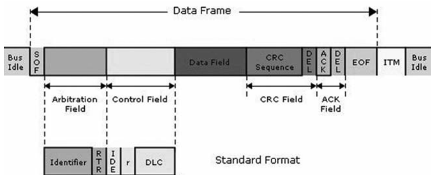
Slika 3.2 – Detaljni prikaz standardne poruke sa podacima
