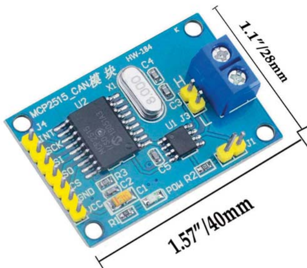
Slika 5.1: Ioumile MCP2515 CAN bus interfejs modul.
