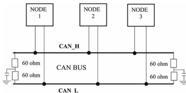
Slika 2.3 – Podjeljeni završetak linije
