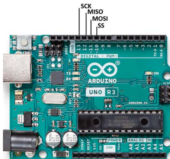
Slika 6.1 – Arduino Uno SPI pinovi
