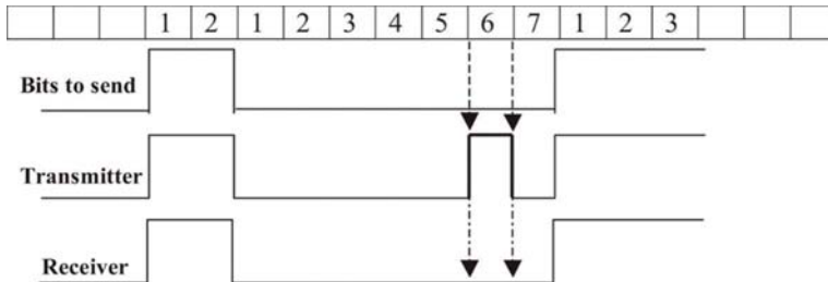
Slika 7.2 - Primer umetanja bita (dodavanje recesivnog bita)
