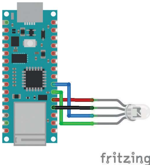
Slika 7-14 Pokrenuti RGB LED sa zajedničkom katodom
