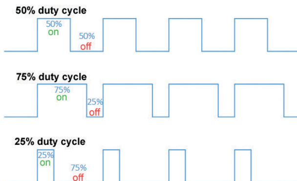
Slika 4-4: Radni ciklus
