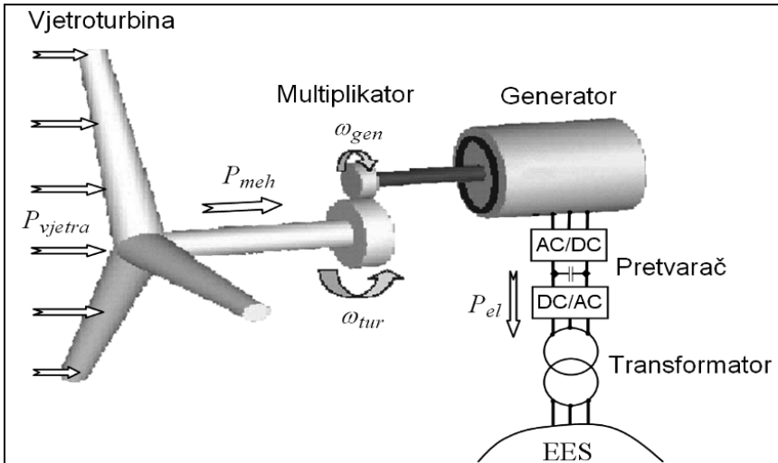
Slika 1.2: Savremeni koncept elektromehaničke konverzije energije vjetra u vjetroagregatima koji su priključeni na EES
